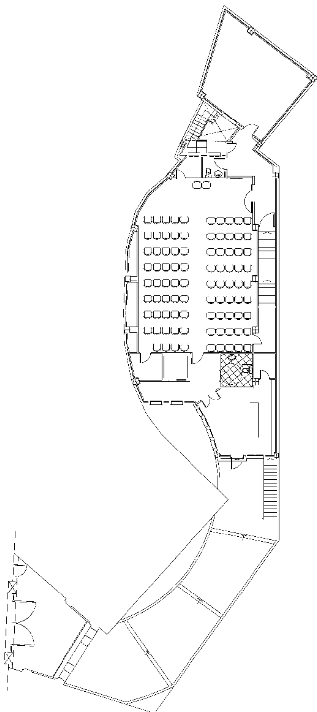
Plano de la primera planta de la nueva Casa Hermandad y Museo de la Soledad
