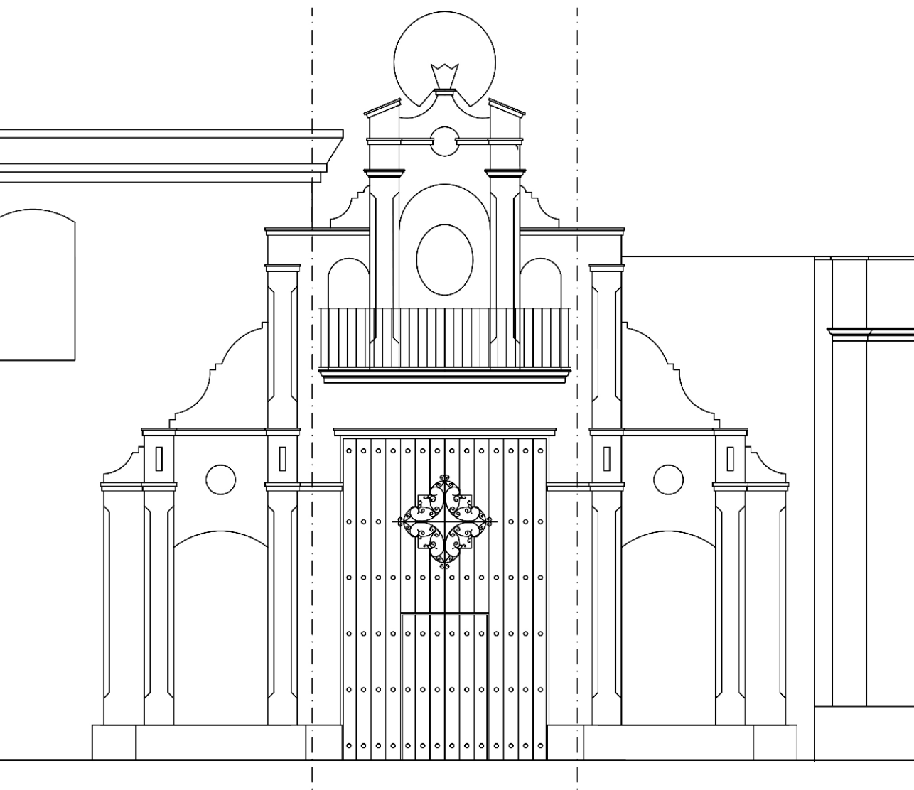
Alzado, en una proyección desplegada, de la planimetría de la fachada principal de la nueva Casa Hermandad y Museo de la Soledad
